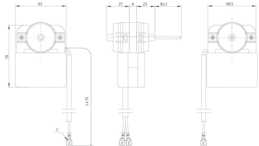
电机性能参数表 Motor performance parameter table
