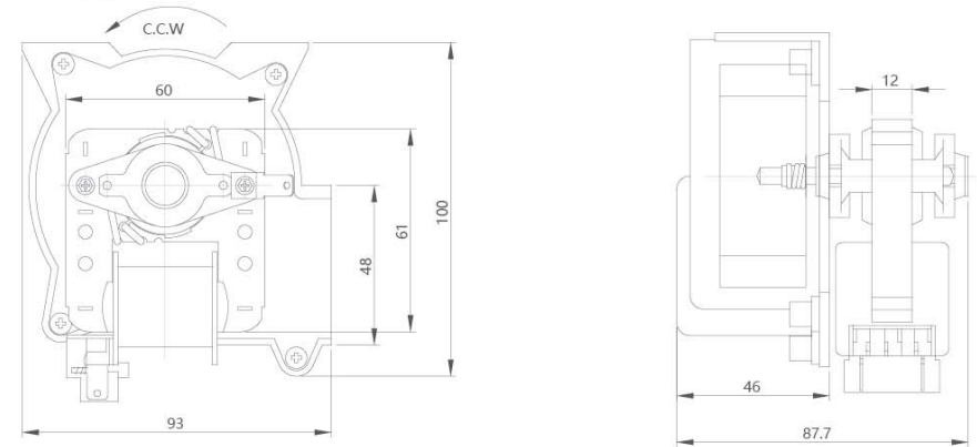
电机性能参数表 Motor performance parameter table
