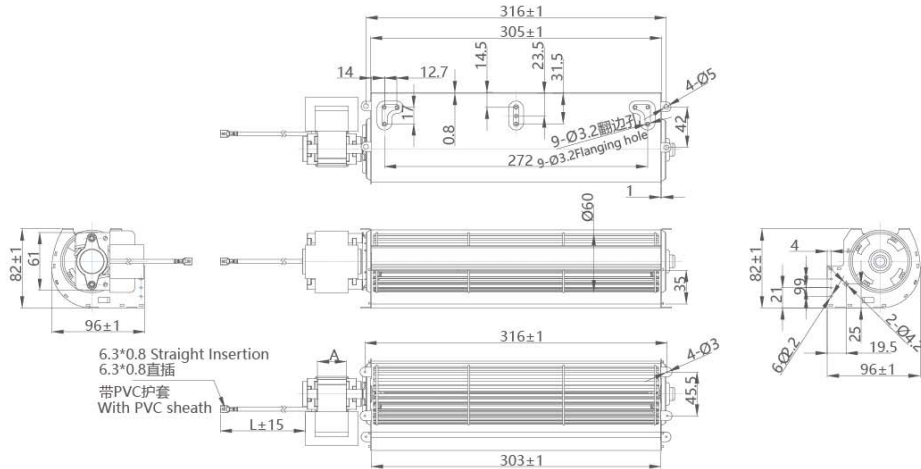
电机性能参数表 Motor performance parameter table
