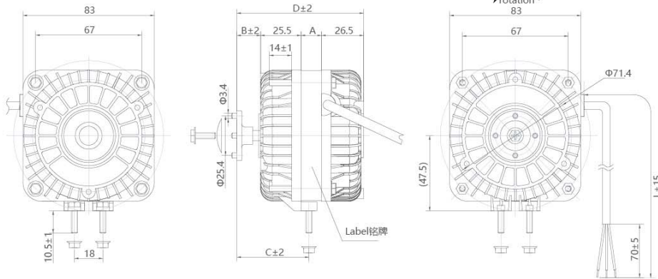
电机性能参数表 Motor performance parameter table
