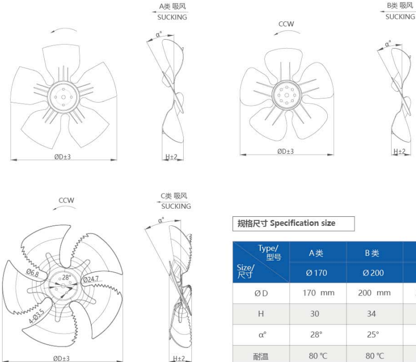
A类风叶 Fan Blade (Type A)
