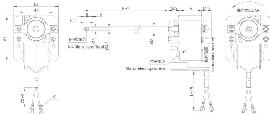
电机性能参数表 Motor performance parameter table
